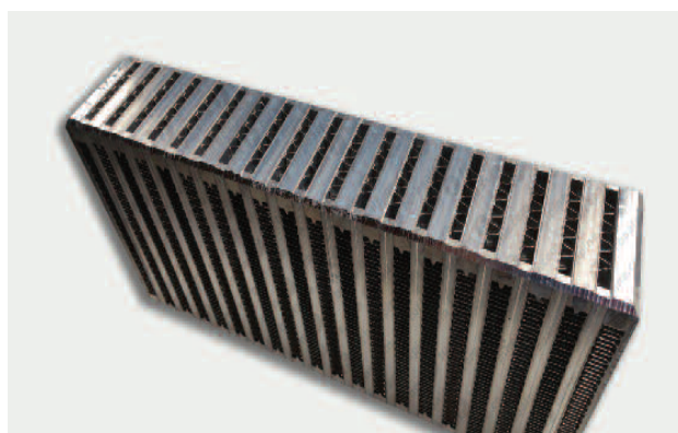
Faisceau style 200 cv Panel estilo 200 cv
