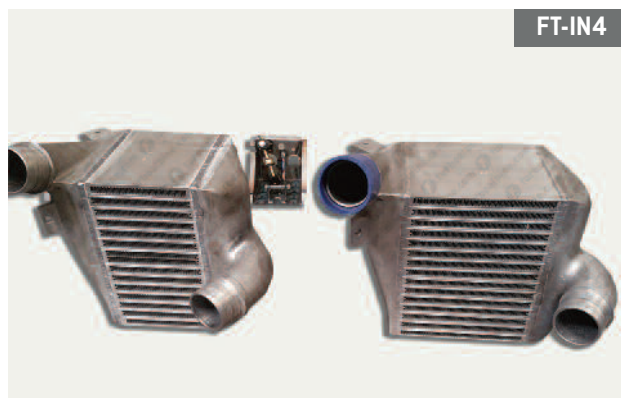
Intercooler TDC sur mesure pour montage alternateur origine Intercooler TDC personalizado para el montaje del alternador original
