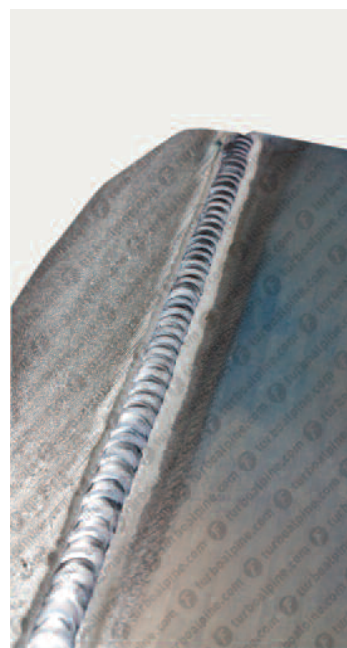
Détail de soudure en aluminium Detalle soldadura en aluminio
