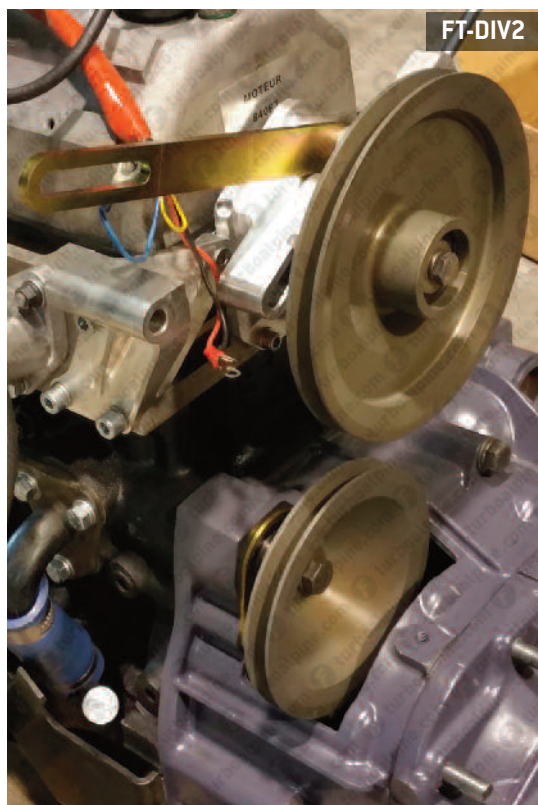
Kit poulies Kit de poleas
