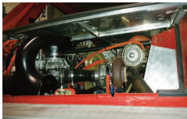
Cache moteur R5 Turbo TDC Cubierta del motor R5 Turbo TDC
